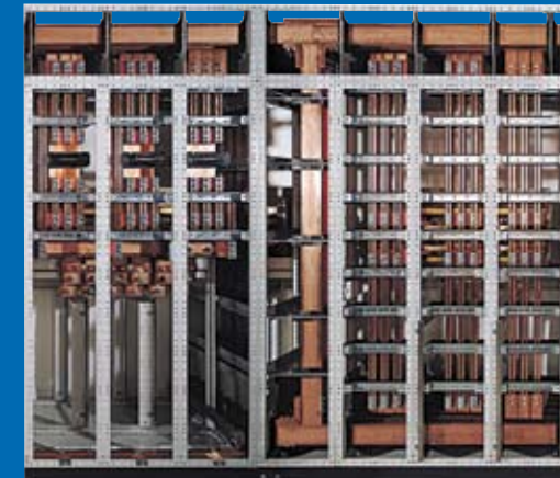
7000A Stromschienensystem mit Hauptschalter in IEC-Applikation
