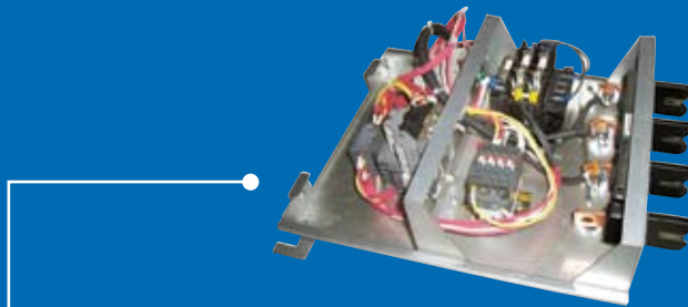
Starter und Motorsteuerung in Einschub- und Auszugstechnik
